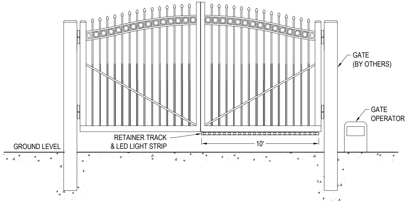
ELEVATION SWINGGATEKIT10 SHOWN
