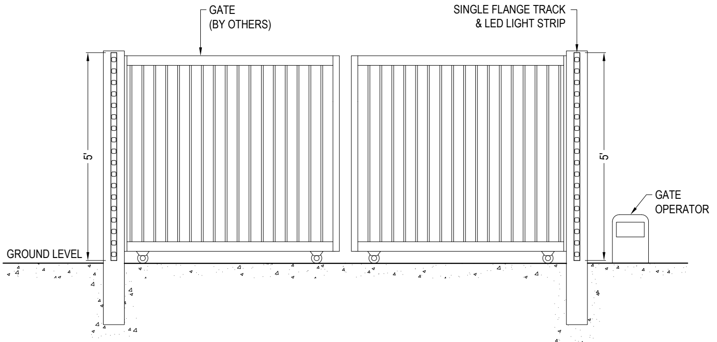
ELEVATION
